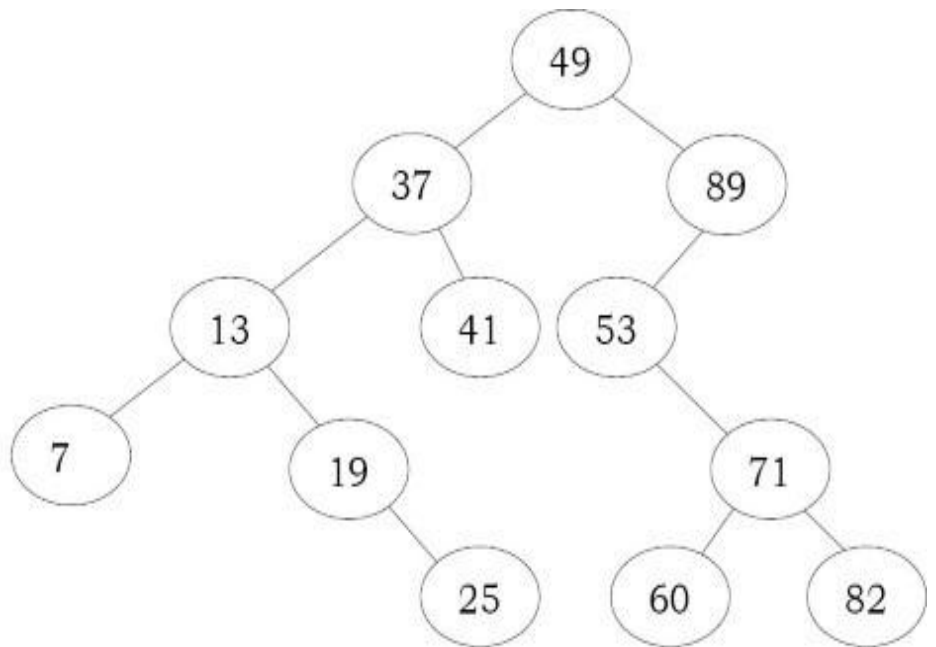
PruneBST(53,79);
