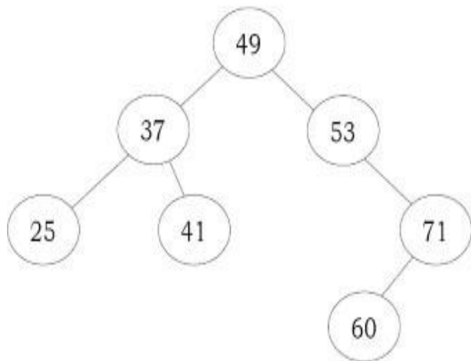
PruneBST(24,71);
