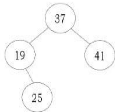
PruneBST(17,41);
