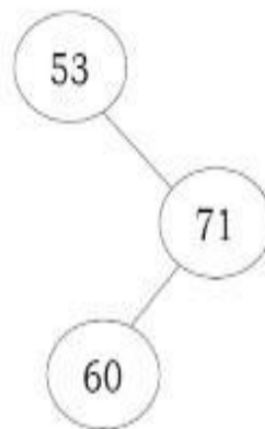
PruneBST(53,79);
